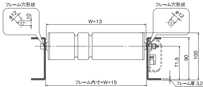
■ フレームセット寸法図
