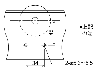
■ フレーム取付穴加工寸法
