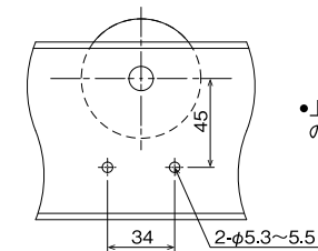
■ フレーム取付穴加工寸法
