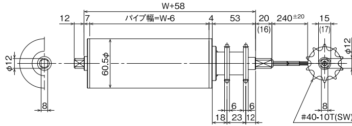
■ モーターローラ寸法図 ※高トルクの場合は( )内寸法となります。
