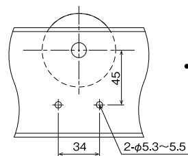
■ フレーム取付穴加工寸法
