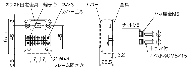
■ 標準付属品 端子台付取付金具 (品番No.AW-001)
